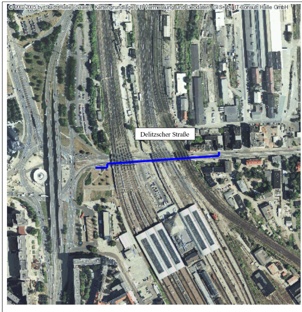
Bild: Baubereich Umverlegung TWL DN 300 Delitzscher Straße vom Riebeckplatz bis Am Güterbahnhof, Hauptbahnhof Halle (Saale) in der unteren Bildhälfte
