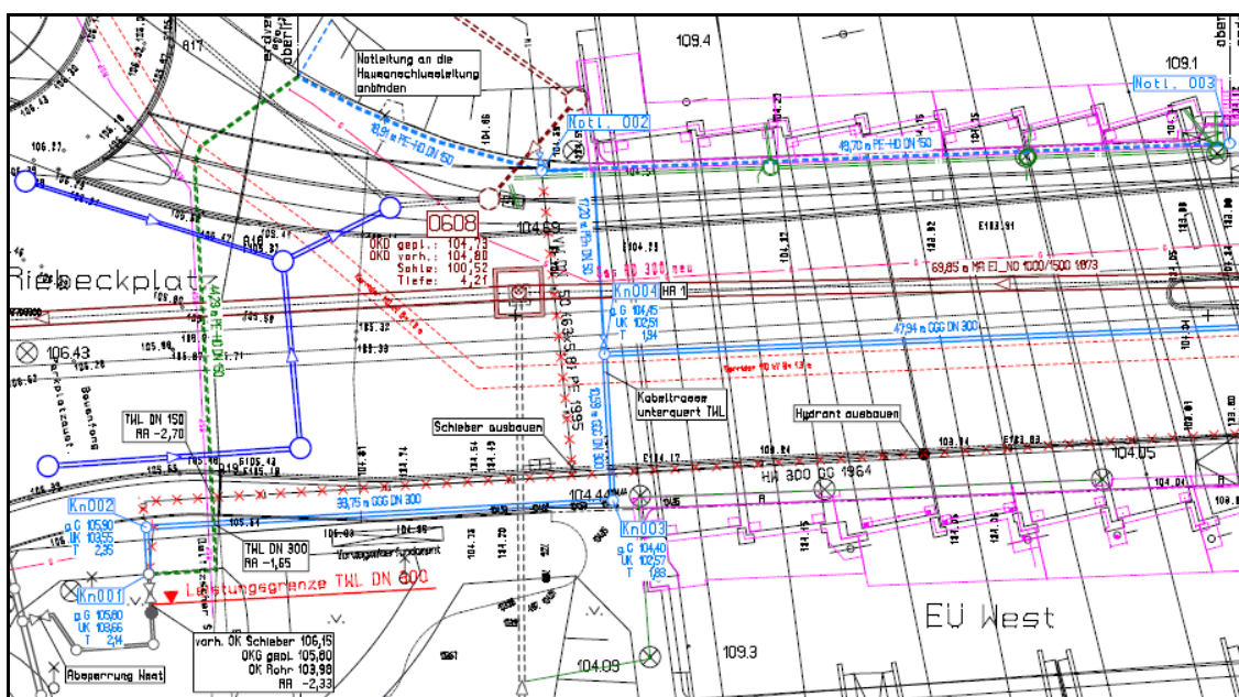
Auszug aus dem Lage- und Absteckplan
